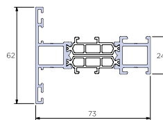
Slim Transom- Cleat Fix ACW81.444
