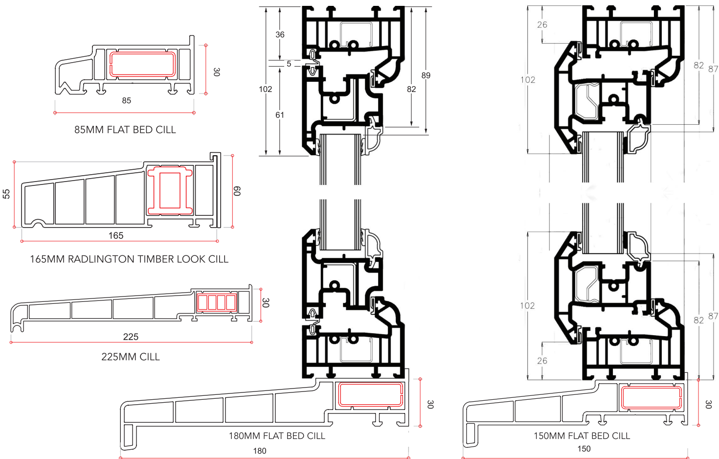
RUSTIQUE O/F WITH FLUSH SASH
