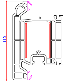
705541 (P10541) Door Sash - Open Out Steel U Channel 713162 (S00162)
