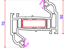
702536 (P10536) 70mm Z Transom Steel Box 713187 (S00167)
