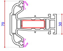
702533 (P10533) 70mm T Transom Steel Box 713187 (S00167)
